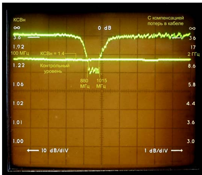
Рисунок 4. Типовая частотная зависимость КСВн антенны АП1-900 с кабельным вводом 30м в диапазоне частот 100-2000 МГц.
