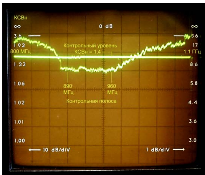
Рисунок 3. Типовая частотная зависимость КСВн антенны АП1-900 с кабельным вводом 30м в диапазоне частот 800-1100 МГц.
