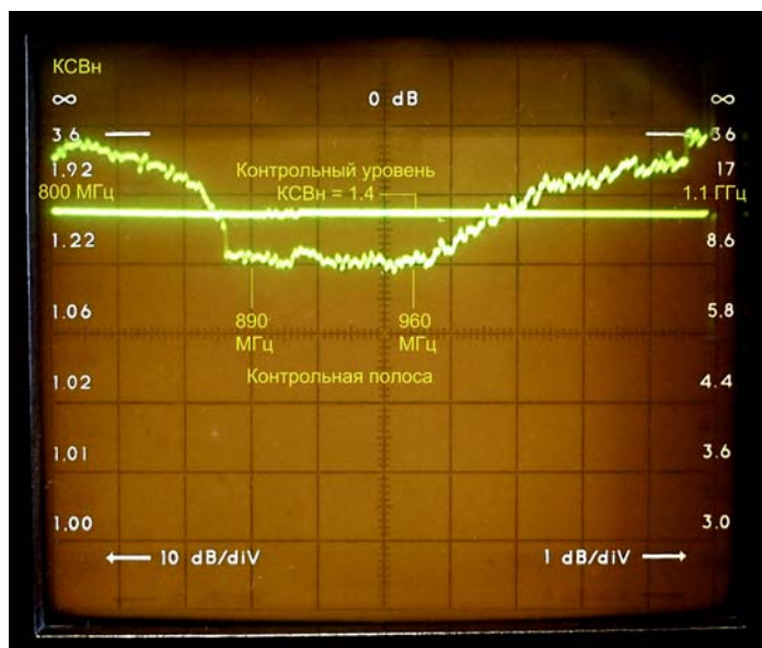
Рисунок 3. Типовая частотная зависимость КСВн антенны АП1-900 с кабельным вводом 25м в диапазоне частот 800-1100 МГц.
