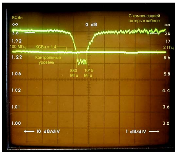
Рисунок 4. Типовая частотная зависимость КСВн антенны АП1-900 с кабельным вводом 25м в диапазоне частот 100-2000 МГц.
