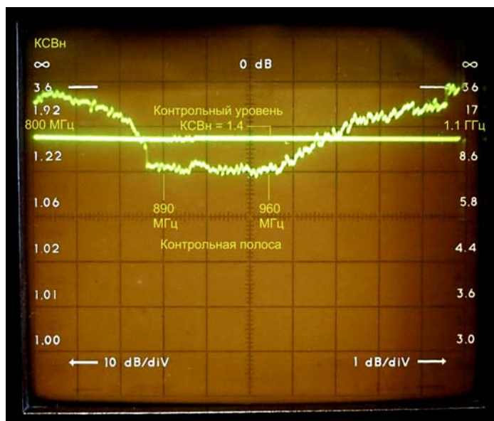
Рисунок 3. Типовая частотная зависимость КСВн антенны АП1-900 с кабельным вводом 20м в диапазоне частот 800-1100 МГц.
