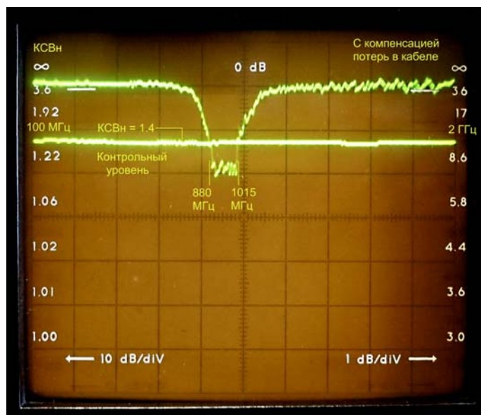
Рисунок 4. Типовая частотная зависимость КСВн антенны АП1-900 с кабельным вводом 20м в диапазоне частот 100-2000 МГц.
