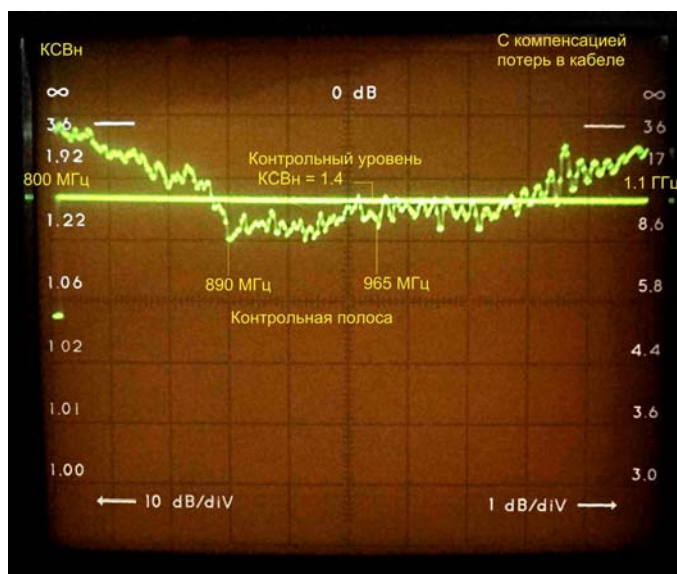
Рисунок 3. Типовая частотная зависимость КСВн антенны АП1-900 с кабельным вводом 15м в диапазоне частот 800-1100 МГц.
