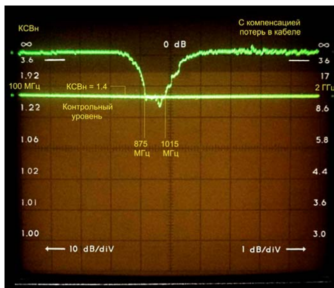
Рисунок 4. Типовая частотная зависимость КСВн антенны АП1-900 с кабельным вводом 15м в диапазоне частот 100-2000 МГц.
