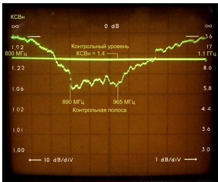
Рисунок 3. Типовая частотная зависимость КСВн антенны АП1-900 с кабельным вводом 10м в диапазоне частот 800-1100 МГц.
