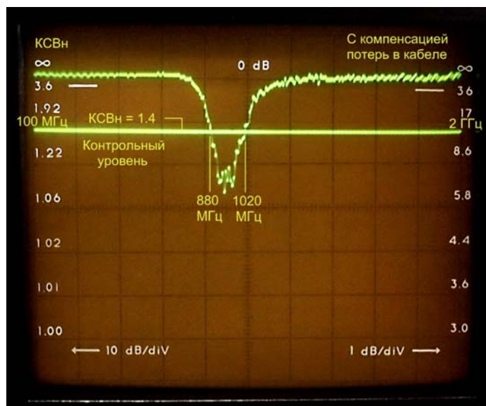
Рисунок 4. Типовая частотная зависимость КСВн антенны АП1-900 с кабельным вводом 10м в диапазоне частот 100-2000 МГц.
